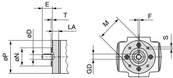
Vierkant-Flansch
